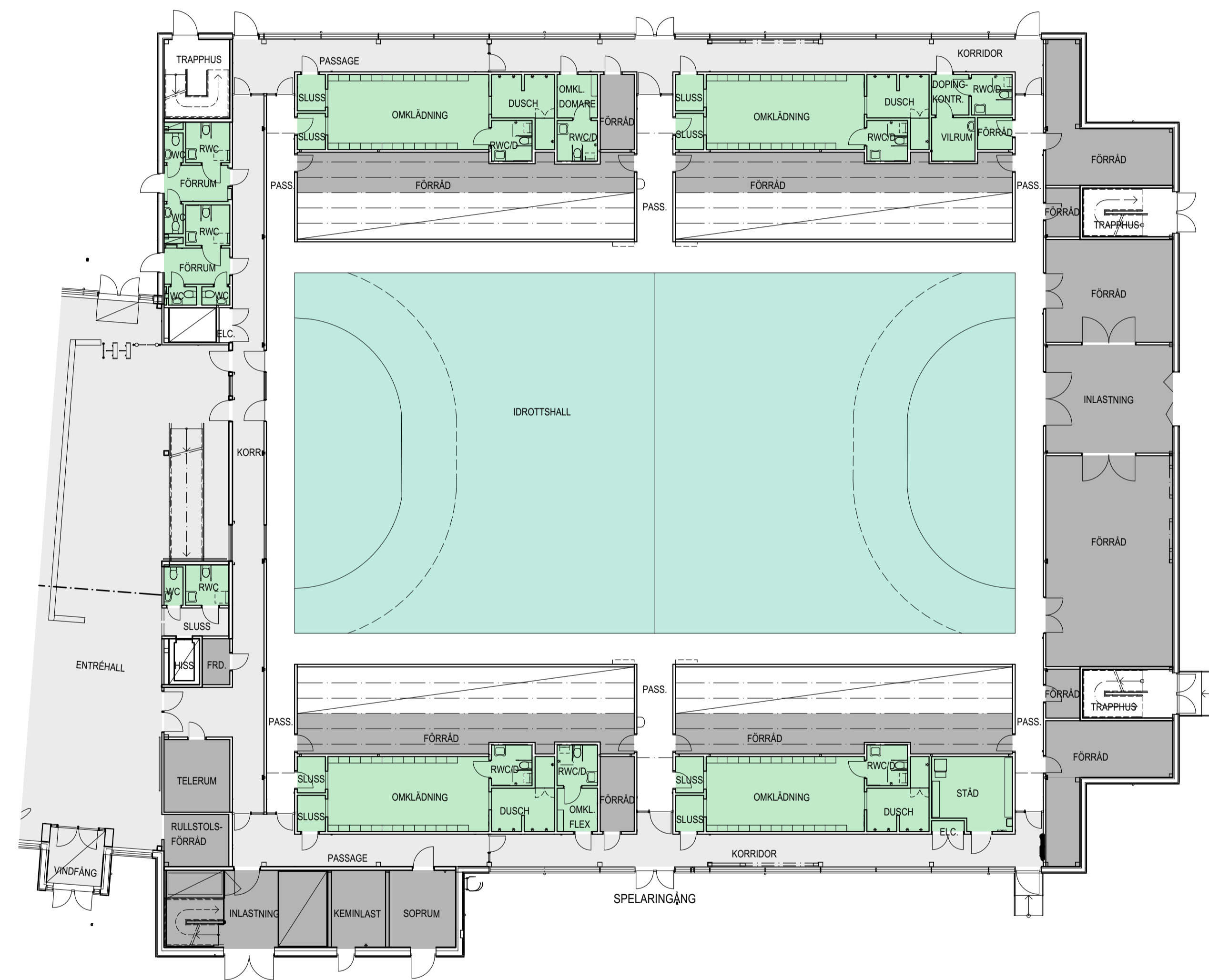
ENTRÉPLAN IDROTTSBALL
