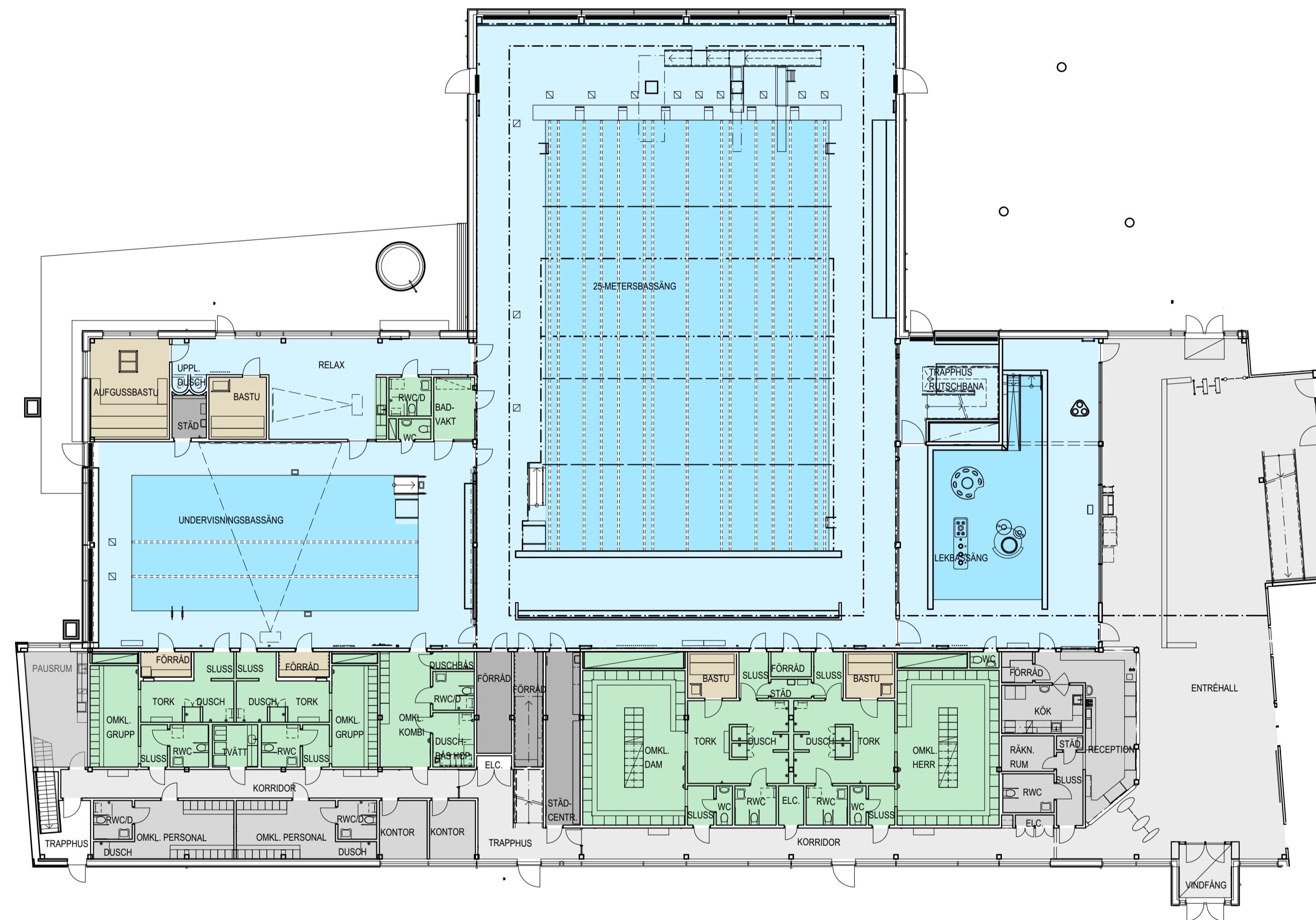
ENTRÉPLAN BADHUS
