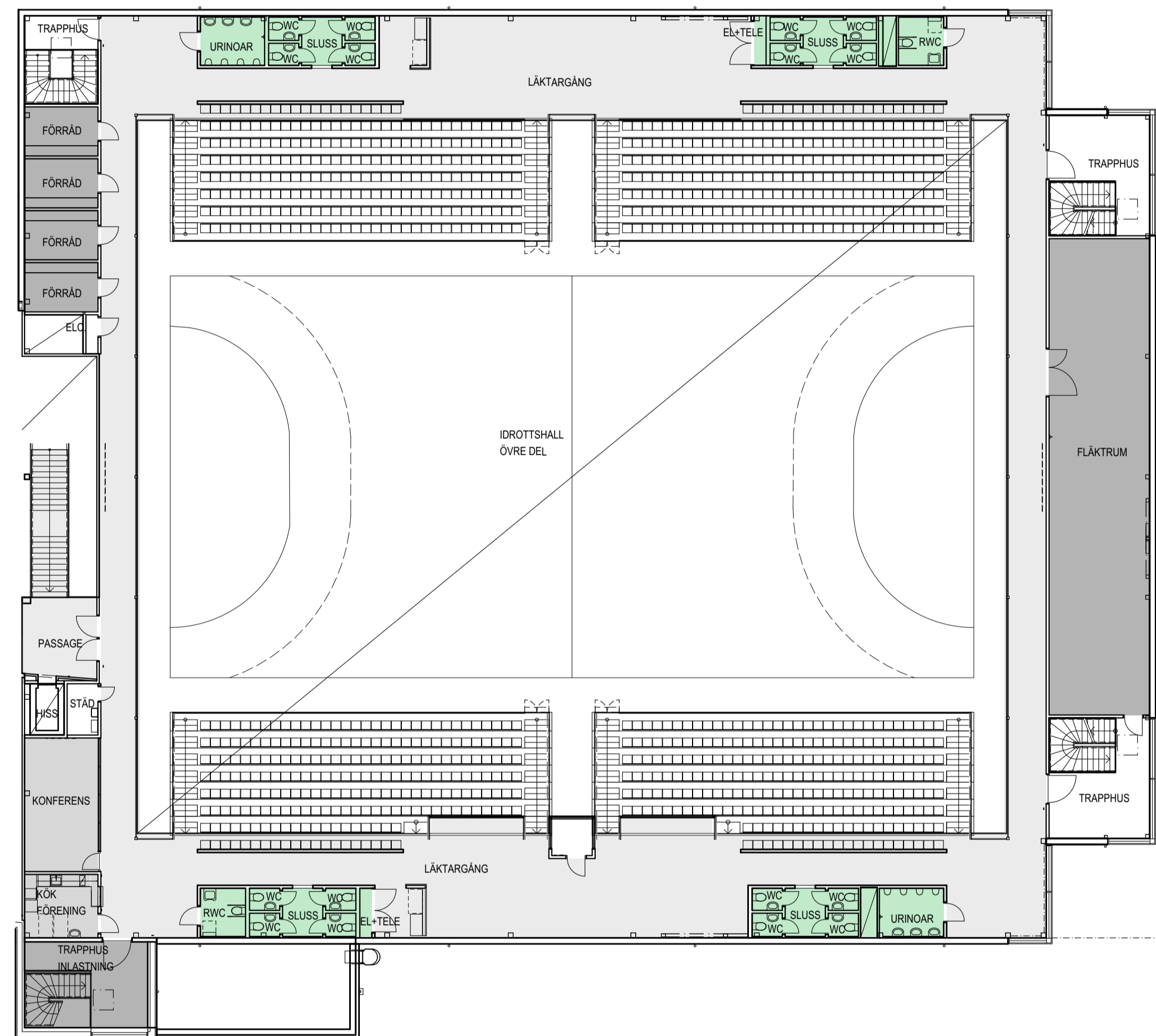
ÖVRE PLAN IDROTTHALL
