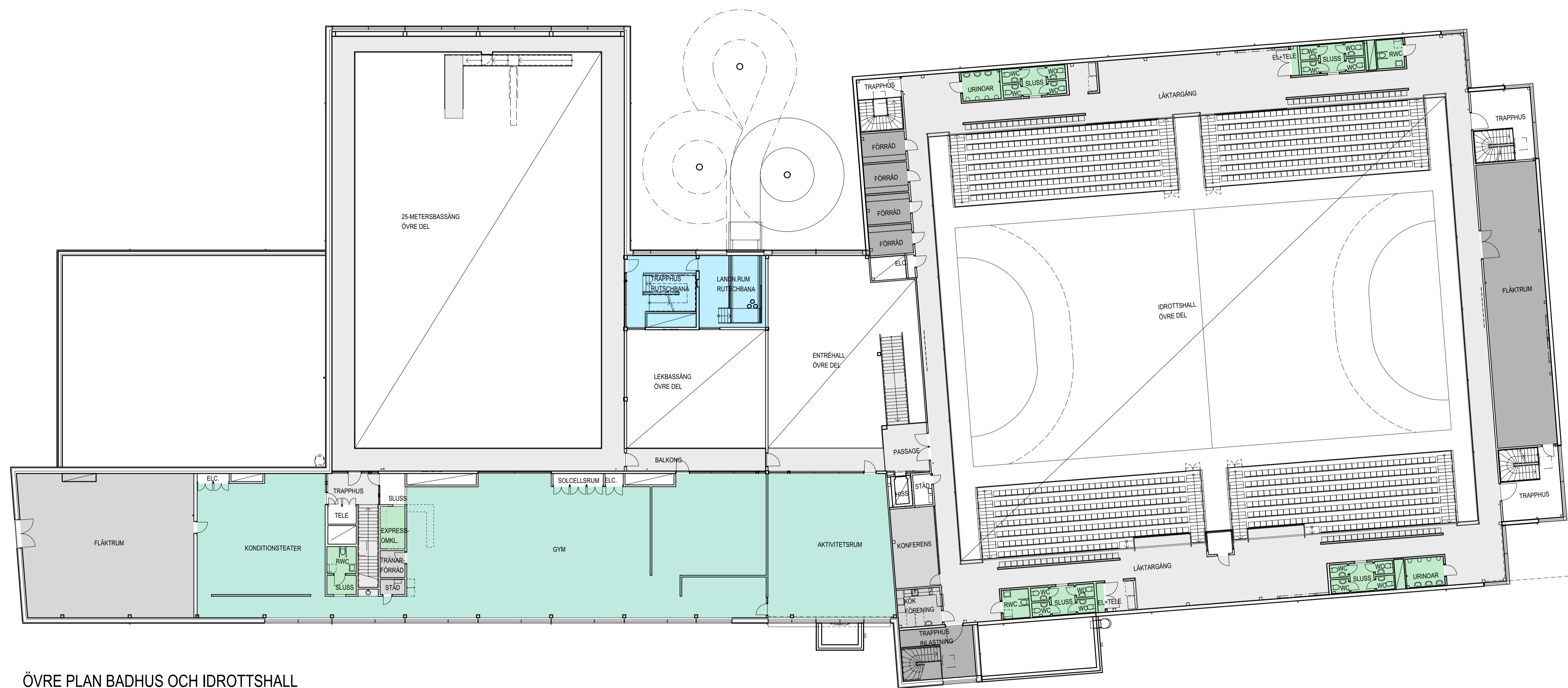
ÖVRE PLAN BADHUS OCH IDROTTSBALL
