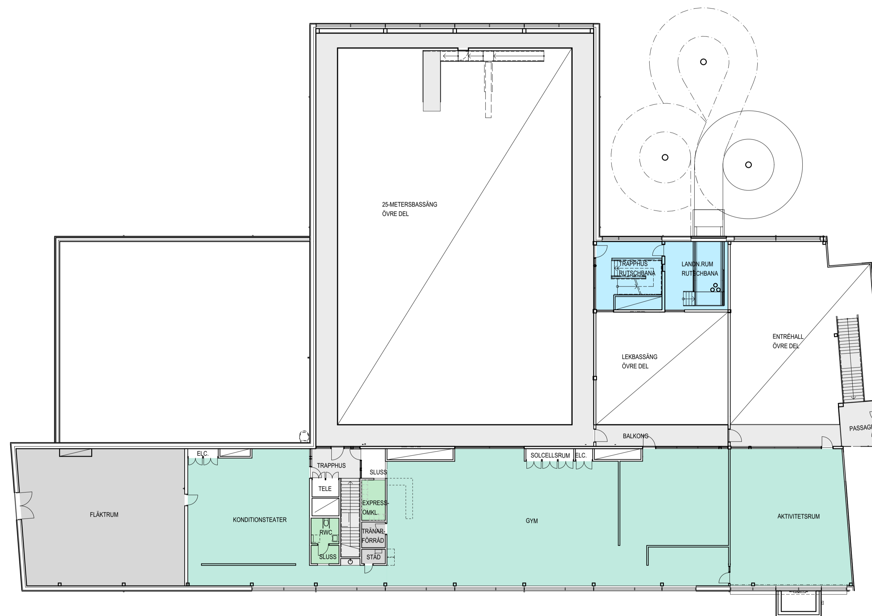
ÖVRE PLAN BADHUS
